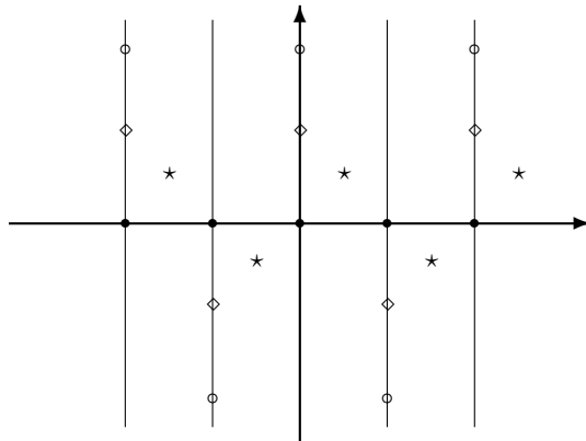
Figura 3.2: Órbitas en la banda de Möbius
