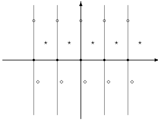
Figura 3.1: Órbitas en un cilindro
