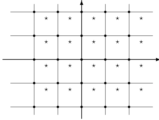
Figura 3.3: Órbitas en un toro
