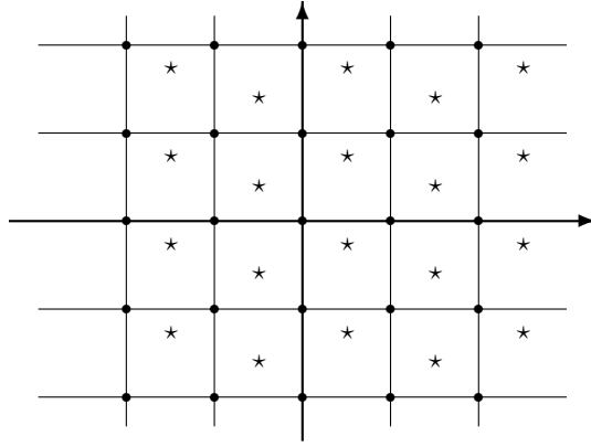
Figura 3.4: Órbitas en una botella de Klein
